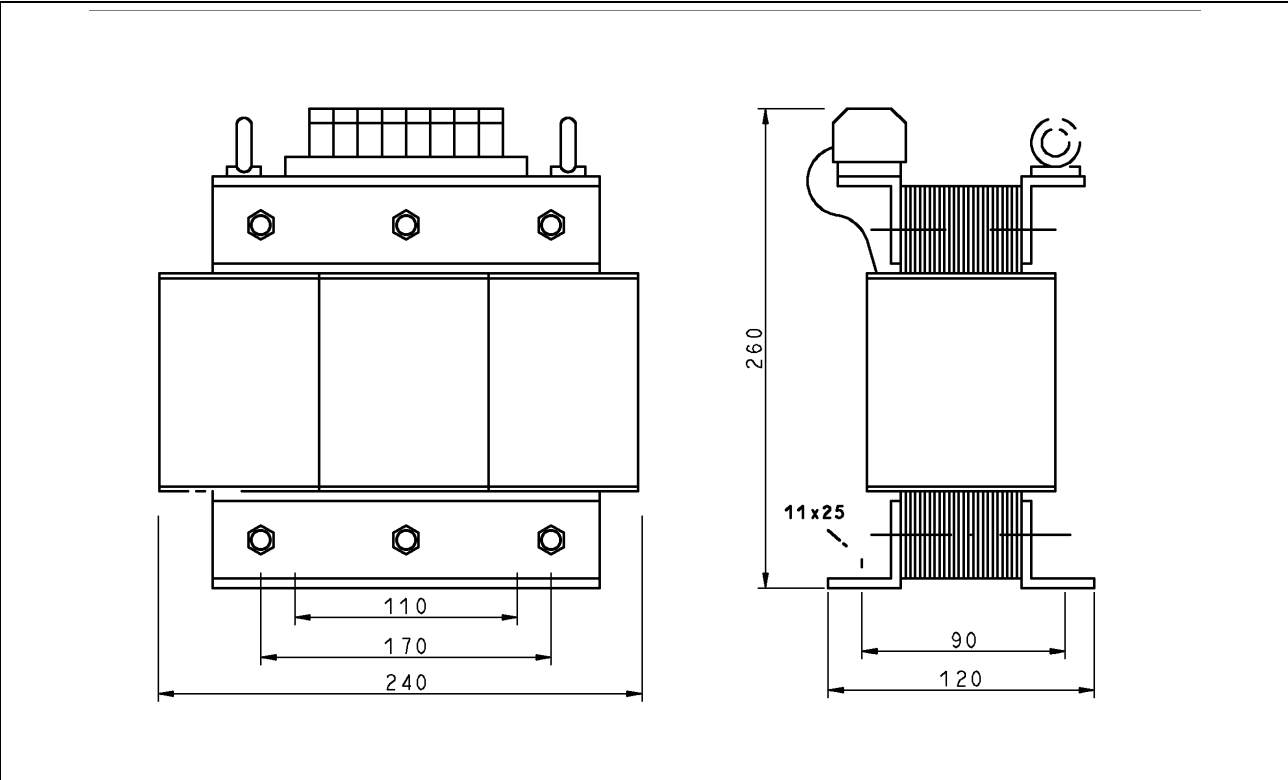
Fig. 10-47: Dimensions
