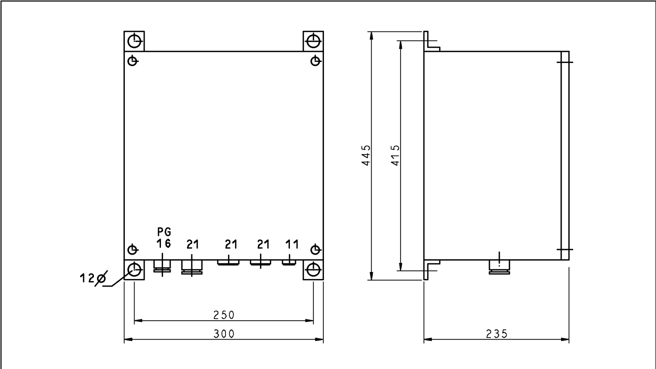
Fig. 10-53: Dimensions
